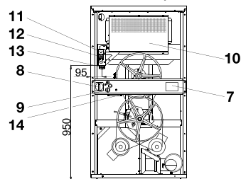
ВИД СЗАДИ T 9 (МОДЕЛЬ С ГАЗОВЫМ НАГРЕВОМ)
