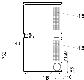
ВИД СЗАДИ T 9 (МОДЕЛЬ С ЭЛЕКТРИЧЕСКИМ НАГРЕВОМ)
